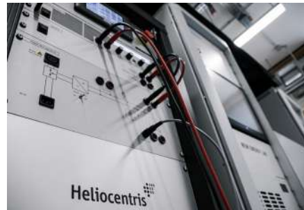
Beispielhafter Versuchsaufbau
